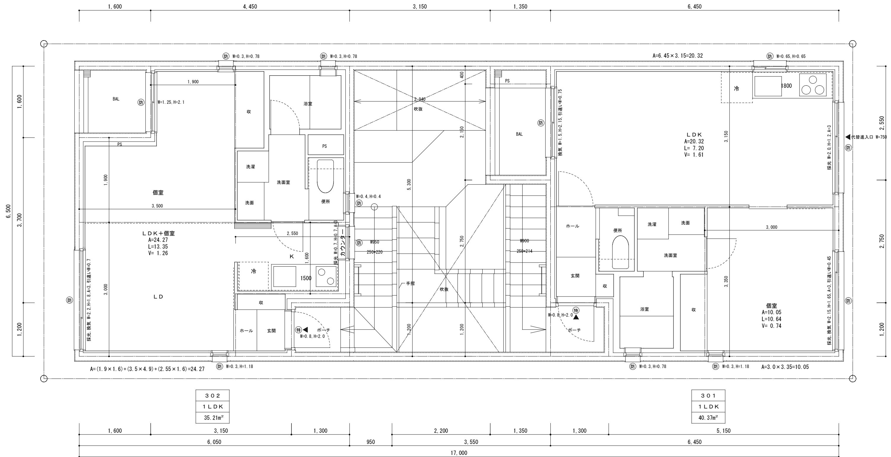
< 3 F 平面図 >
